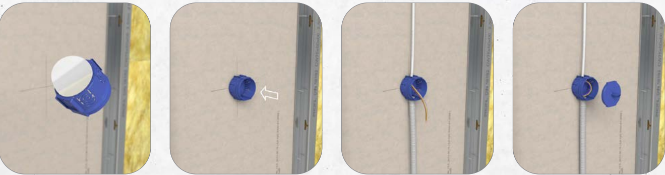
1. Klebescheibe (P005) auf die Unterseite der Multidose (P002) aufkleben und die Folie abziehen. 2. Dose an gewünschter Stelle aufkleben. 3. Leitungen und Rohre einführen. 4. Bohrdeckel (P003) aufsetzen.
