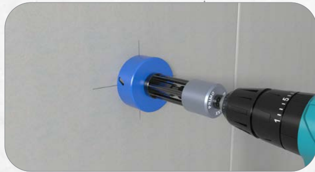
1. Erste Dose anzeichnen und mit PRIMO Bohr-Fixx (P779) und 74 mm Lochsäge (P797-74) von der Vorderseite ausbohren.
