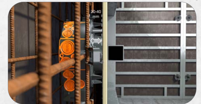
4. Flexible Flügel (P761) passen sich der jeweiligen Betonbedeckung an. Betonbedeckungen zwischen 20 – 40 mm oder 40 – 60 mm sind möglich. Nach dem Stellen der Gegenschalung kann betoniert werden.
