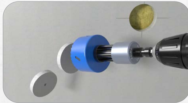
2. Einfaches Entfernen der Bohrkerne durch Bohr-Fixx (P779).
