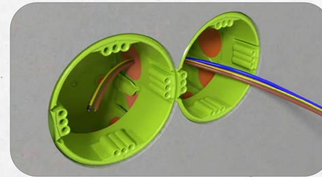
8. Einfache und zeitsparende Durchverdrahtung dank großflächiger Verbindungsmembran.
