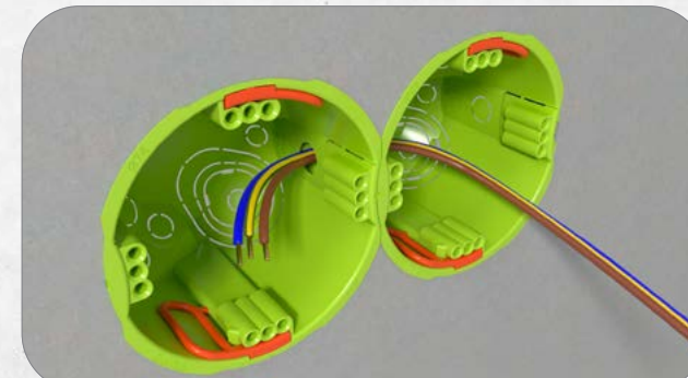
9. Einfache und zeitsparende Durchverdrahtung dank großflächiger Ausbrechöffnung möglich.
