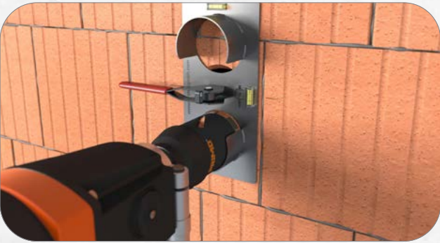
1. Erste Dose anzeichnen und mit 82 mm Bohrkronen ausbohren. Für Mehrfachkombinationen Unterputzbohrschablone (P718) verwenden.
