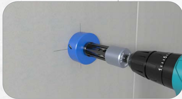
1. Erste Dose anzeichnen und ein 74 mm Bohrloch einbringen.
