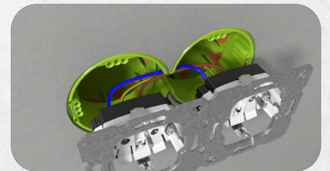
11. Einfache Installation vorverdrahteter Geräte durch SCS-Verbindungstechnik.
