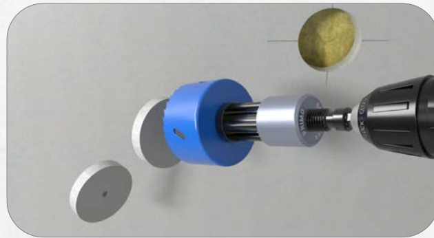
2. Einfaches Entfernen der Bohrkerns durch automatischen Auswurf des Bohrkerns mit Bohr-Fixx (P779).
