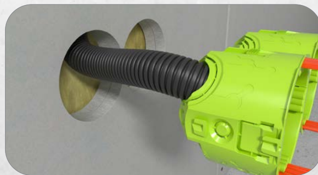
6. Rohr einführen, durch die Ausbrechöffnung wird das Rohr sicher fixiert.
