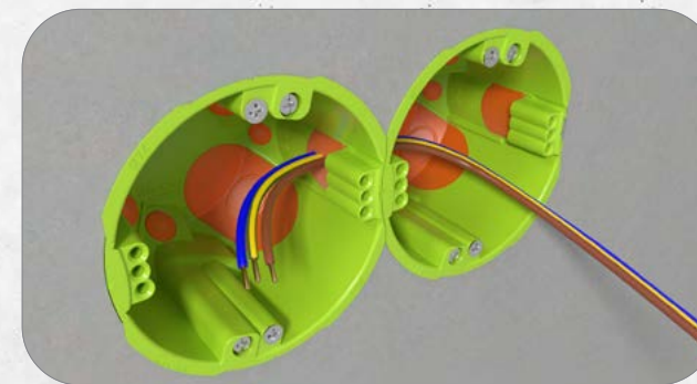
7. Einfache und zeitsparende Durchverdrahtung dank großflächiger Verbindungsmembran.
