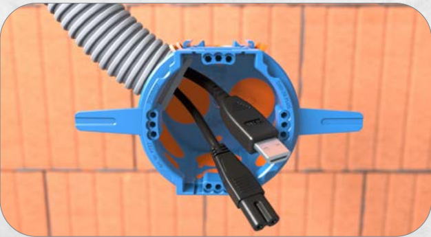
5. Kabel einfach durch Cable-Plopp durchstecken oder Membrane mit Cuttermesser öffnen und Rohre einführen. Vorkonfektionierte Leitungen durch Großrohreinführung M32 installierbar.
