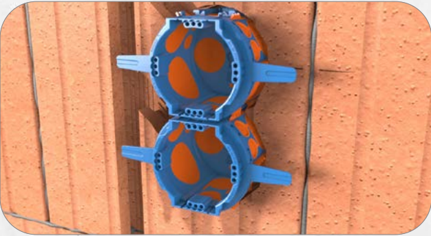
3. Thermodosen mit 71 mm Kombinationsabstand fest verbinden und ins Bohrloch einsetzen. Garantiert putzbündig dank Putzanschlag.
