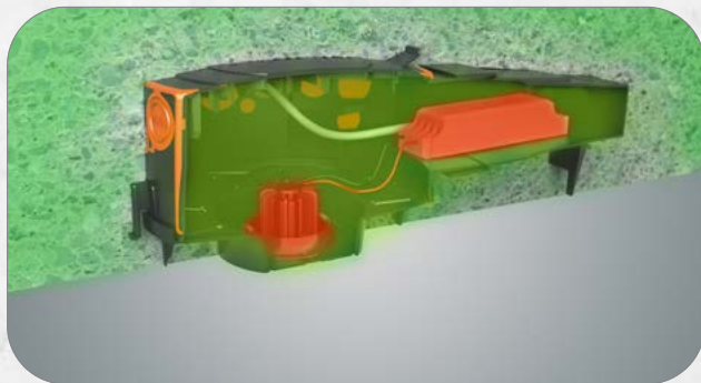
9. Das ideale Thermomanagement im Einbaugehäuse garantiert eine optimale Luftzirkulation. Dies verhindert Hitzestau im Gerät, auch bei Verwendung des zusätzlichen Trafotunnels (P873).
