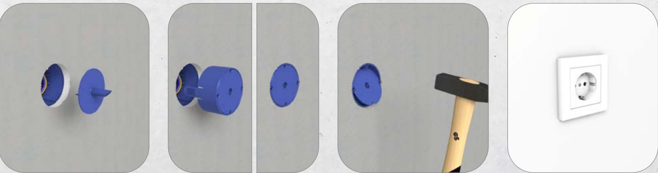
9. Bohrdeckel (P003) entfernen. 10. Dosenoberteil aufstecken und bündig mit der Gipskartonplatte eindücken. 11. Deckel mit einem Hammer ausbrechen. 12. Installation abschließen.
