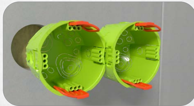
4. Vor dem Einsetzen die Dosen durch die stabile SCS-Verbindungstechnik miteinander verbinden.
