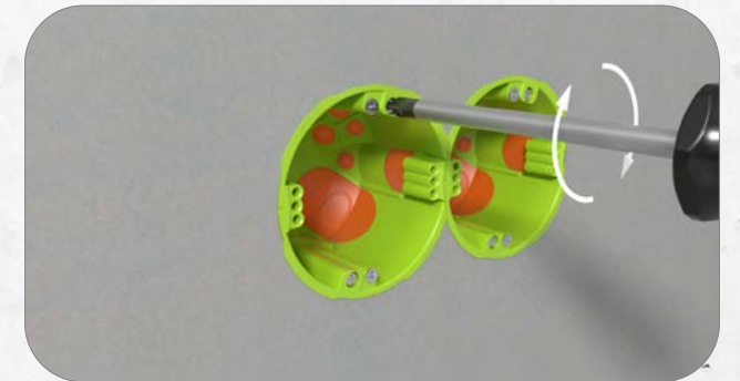
6. Dosen einsetzen und festschrauben.
