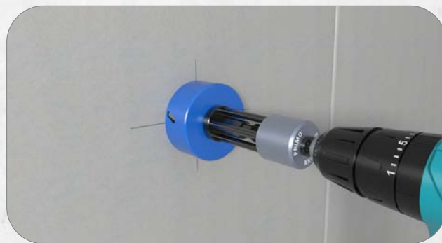
1. Erste Dose anzeichnen und mit PRIMO Bohr-Fixx (P779) und 74 mm Lochsäge (P797-74) ausbohren.
