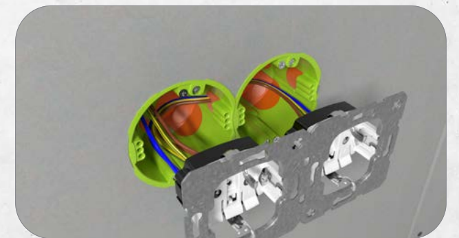
8. Großer Klemmraum ermöglicht einfaches Verdrahten der Geräte.
