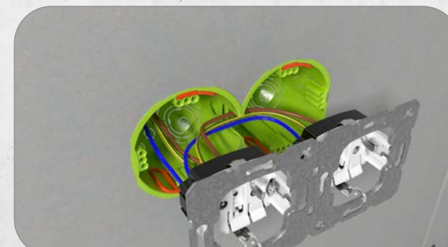
11. Vorverdrahtete Geräte können ganz einfach eingesetzt werden.
