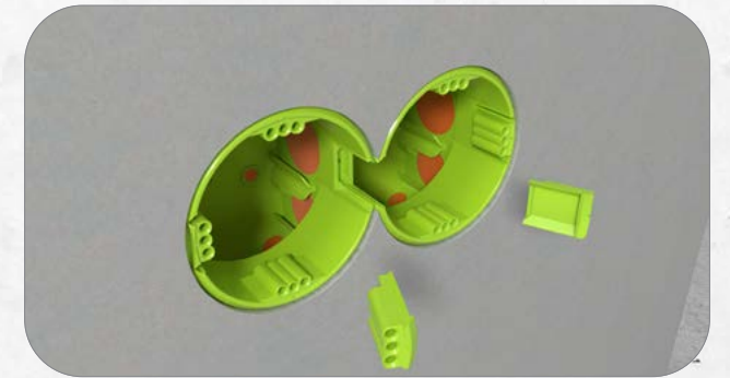
9. Bei Bedarf kann der SCS-Verbindungssteg ausgebrochen werden.
