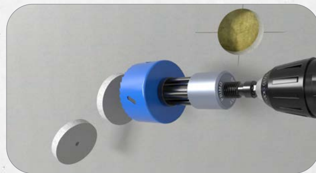
2. Einfaches Entfernen der Bohrkerne durch automatischen Auswurf des Bohrkerns mit Bohr-Fixx (P779).
