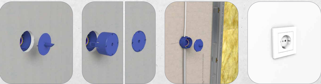
9. Bohrdeckel (P003) entfernen. 10. Dosenoberteil aufstecken und bündig mit der Gipskartonplatte eindrücken. 11. Deckel mit einem Hammer ausbrechen. 12. Installation abschließen.
