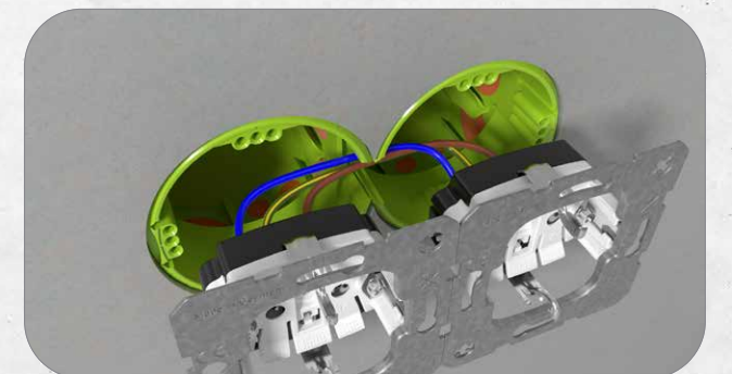
11. Einfache Installation vorverdrahteter Geräte durch SCS-Verbindungstechnik.
