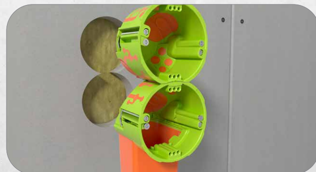
4. Stabile Verbindung durch SCS-Verbindungstechnik.
