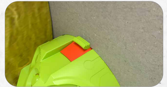
8. Klick-System: Durch das Einschieben der Keile wird die Dose in der Rigips-Platte fixiert.
