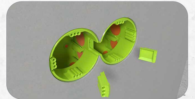
9. Bei Bedarf kann der SCS-Verbindungssteg ausgebrochen werden.
