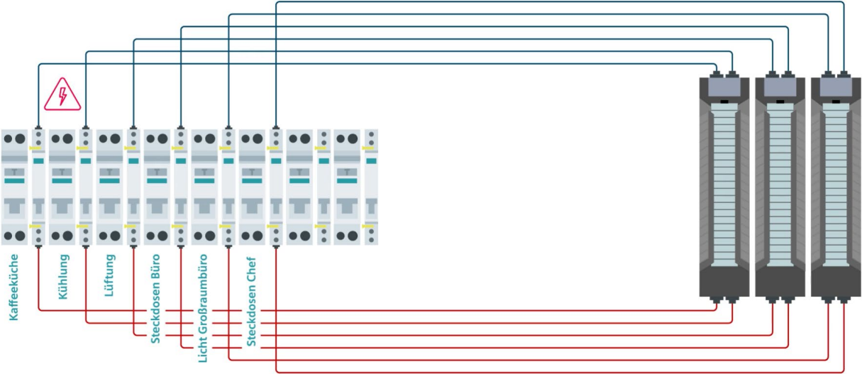
8 Endstromkreise (12TE)
